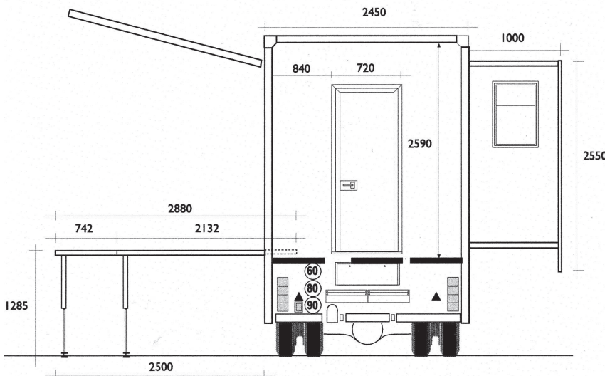
VUE ARRIÈRE
