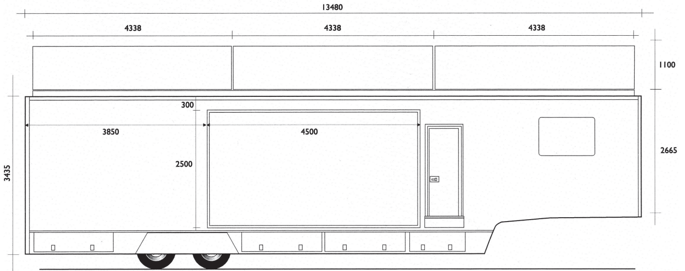
CÔTÉ DROIT
